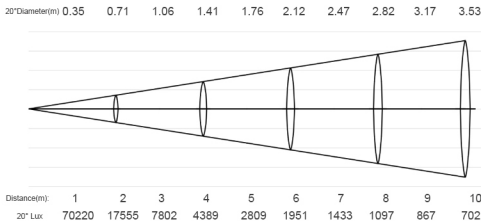
Optical parameters
